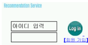
그림 6. 로그인
