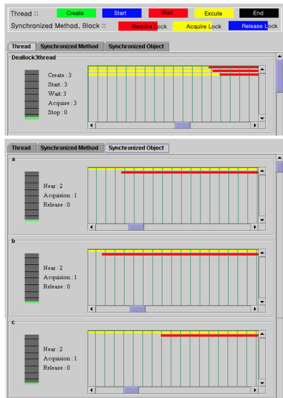
(그림 8) 예제 프로그램의 트레이스
