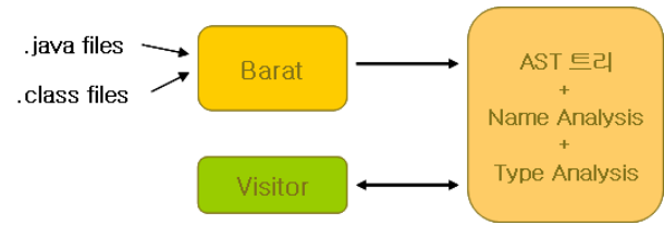
(그림 4) Barat의 구조
